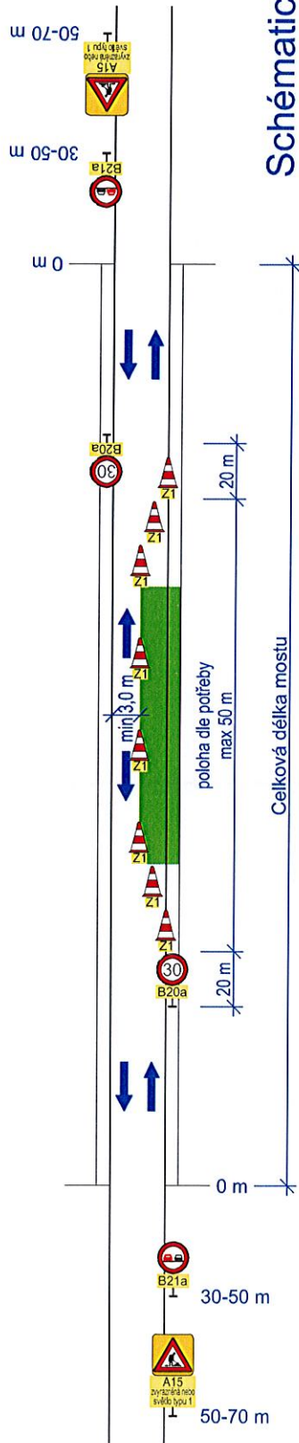
Schéma 1 - pracovní místo na mostě v obci
