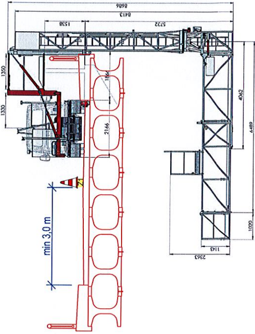
Schématický příčný řez
